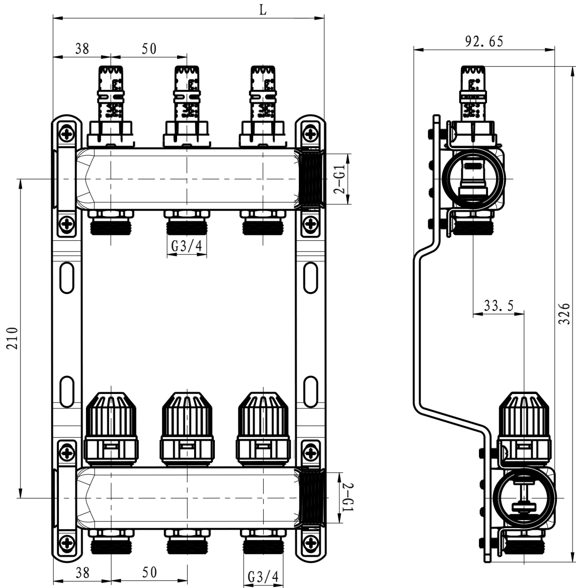
Fußbodenheizungsverteiler
