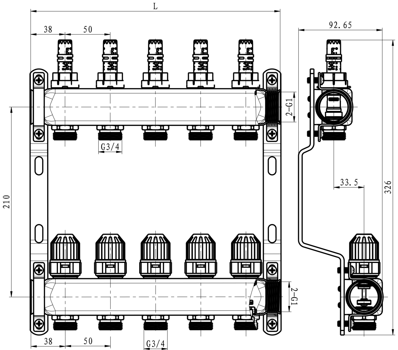
Fußbodenheizungsverteiler
